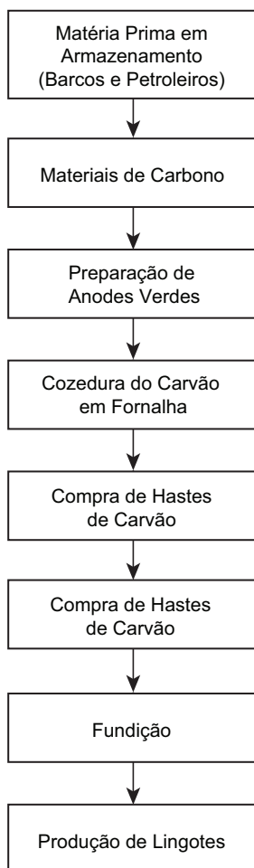
FIGURA 16.2. Processo de produção da Mozal Aluminium.
