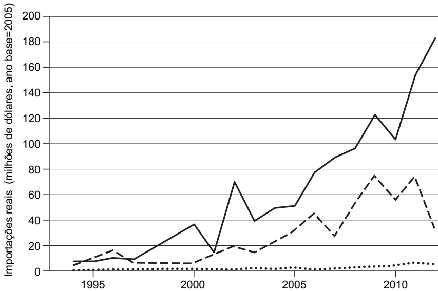
FIGURA 13.3. Importações de Moçambique de materiais de construção (linha contínua, ferro e aço; linha tracejada, cimento; linha pontuada, vidro). (Fonte: UN Comtrade.)
